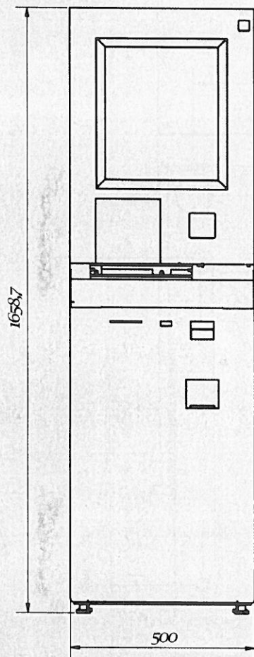
Čelní kótovaný pohled
